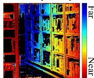
Depth Map
